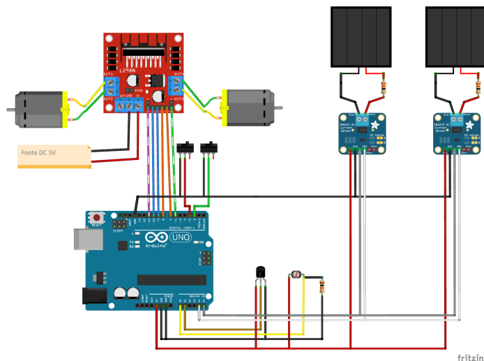
Figure 3: Diagrama de conexões elétricas e esquemático de montagem física dos componentes eletrônicos do ASCM.
