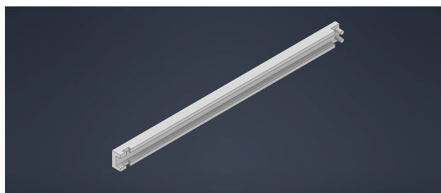
Figure 6: Modelo tridimensional do suporte do rodo motorizado (Wiper Support) e acoplamento do motor com o pinhão.
