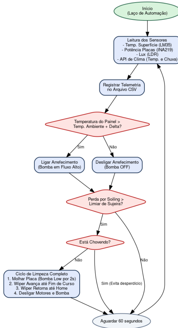
Figure 7: Fluxograma do laço de controle de automação e de tomada de decisão do sistema ASCM.
