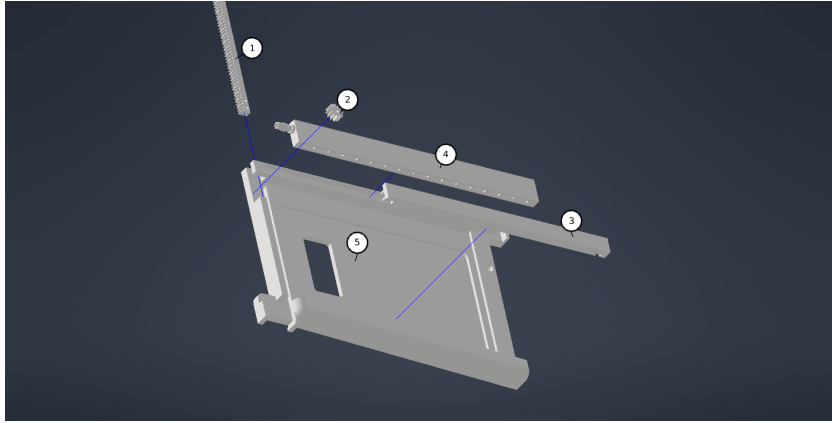
Figura 2: Vista explodida da montagem do mecanismo de translação do ASCM: (1) Cremalheira ( Gear-Rack ); (2) Pinhão ( Gear ); (3) Suporte do Rodo ( Wiper Support ); (4) Suporte de Aspersão ( Sprinkler ); (5) Suporte dos Painéis ( Panel Support ). Fonte: Elaborado pelos autores.
