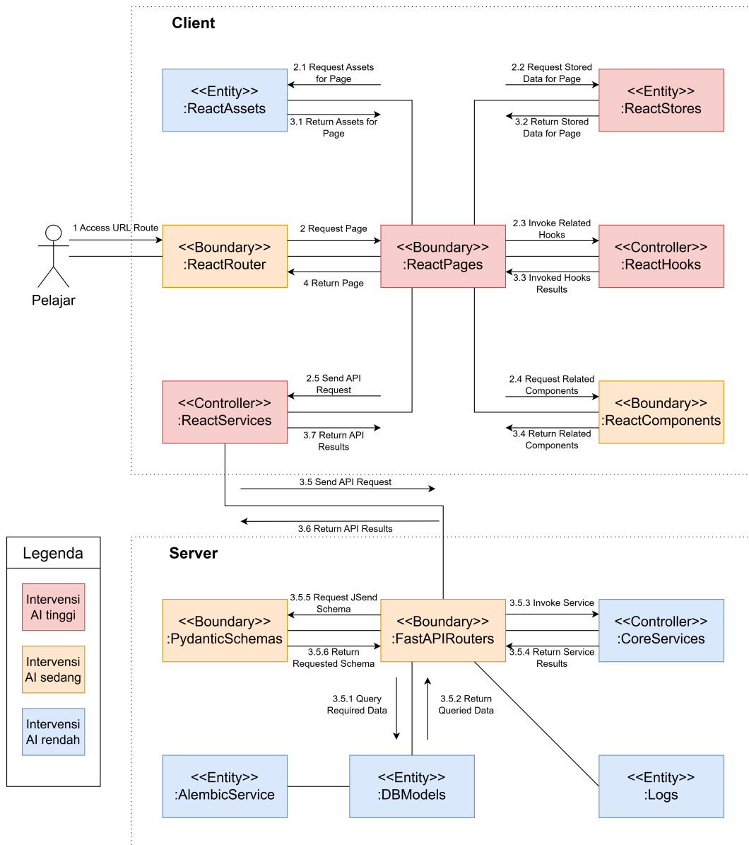
Gambar V.1 Diagram arsitektur client-server untuk Equilibria
