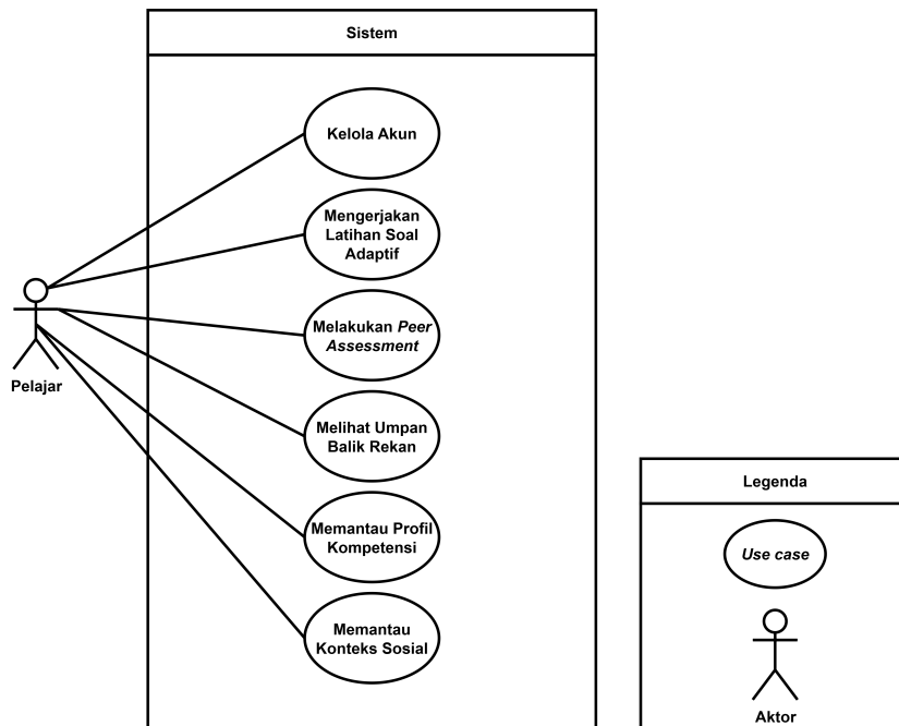
Gambar IV.1 Use Case Diagram - Interaksi pelajar dengan Sistem Asesmen Adaptif Kolaboratif
