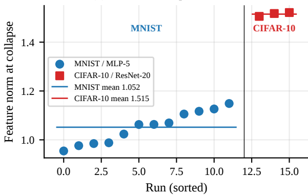
(d) Architecture-specific threshold
