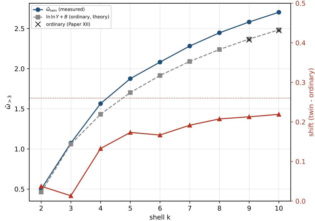
(D) \bar{\omega} drift: main + Mertens B + shift \rightarrow 0.2604
