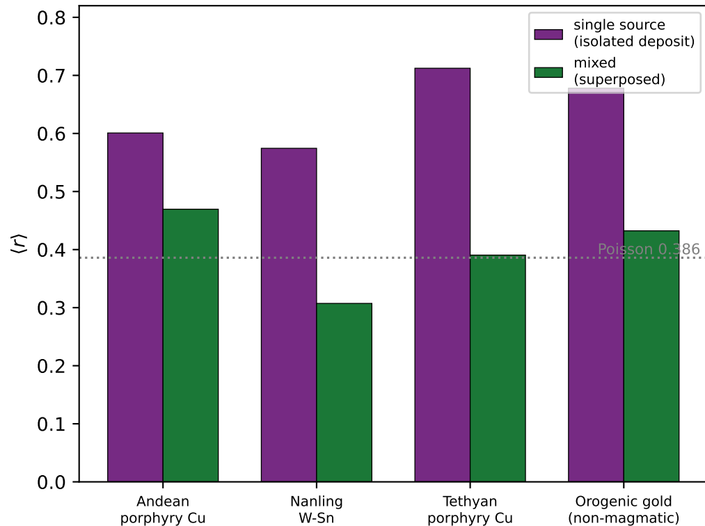
(d) superposition \rightarrow Poisson (retained, real)
