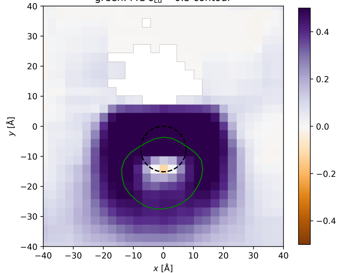
(d) Warren-Cowley \alpha_1 ( 7 \times 7 window) green: MC c_{\text{Lu}} = 0.5 contour
