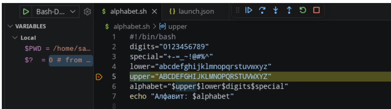
Рисунок 23 – содержимое скрипта alphabet.sh с возможностью установки точки остановки
