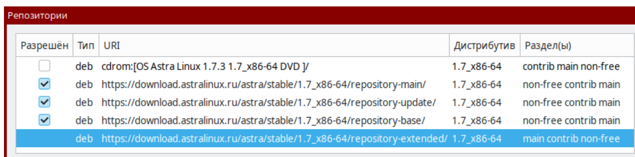
Рисунок 30 – окно настройки репозитриев Synaptic со снятой галочкой напротив extended-репозитория
