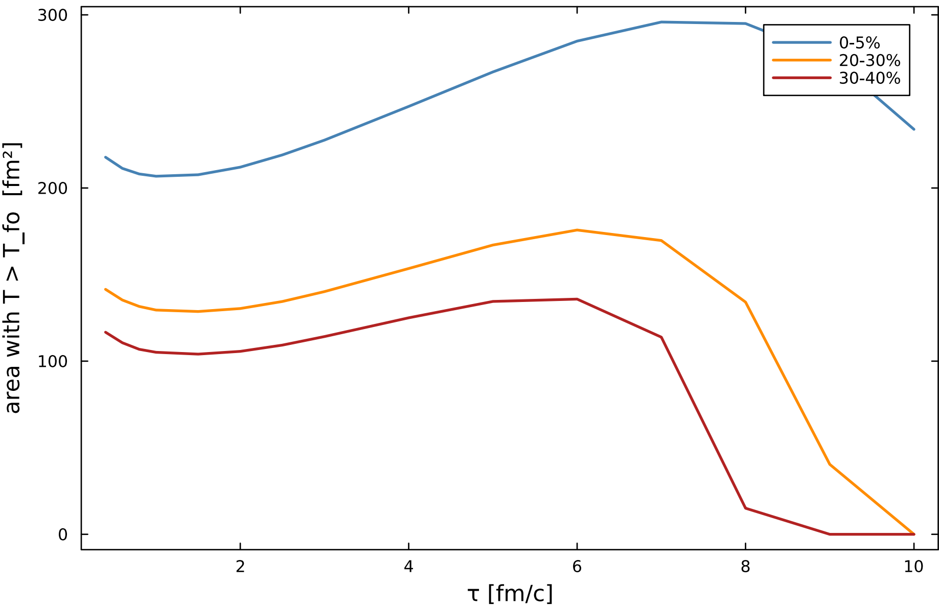
Fireball lifetime ( T_{fo} = 0.1565 GeV)
