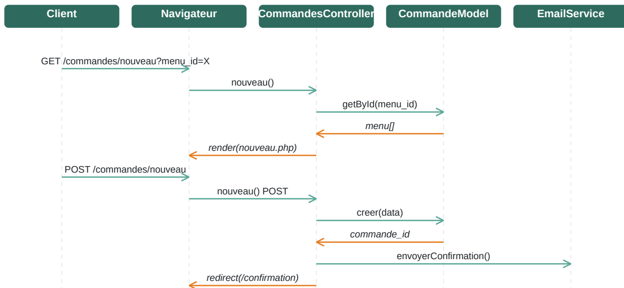
Diagramme de séquence — Commande
