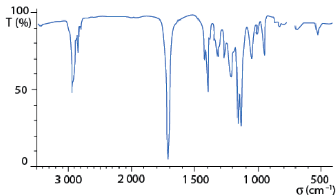
Document 2: Spectres IR à attribuer
