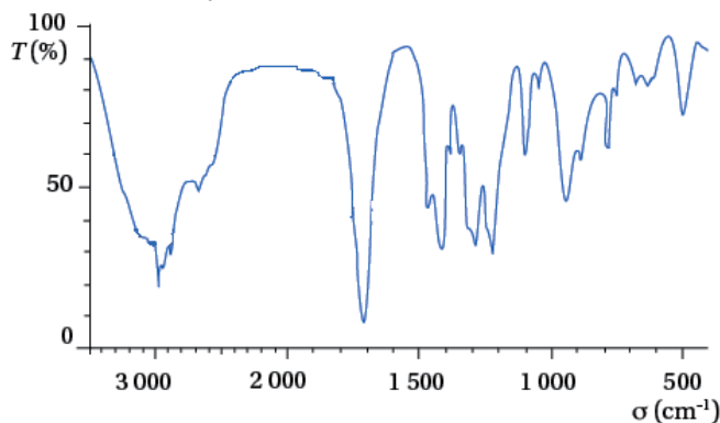
Document 2: Spectres IR à attribuer
