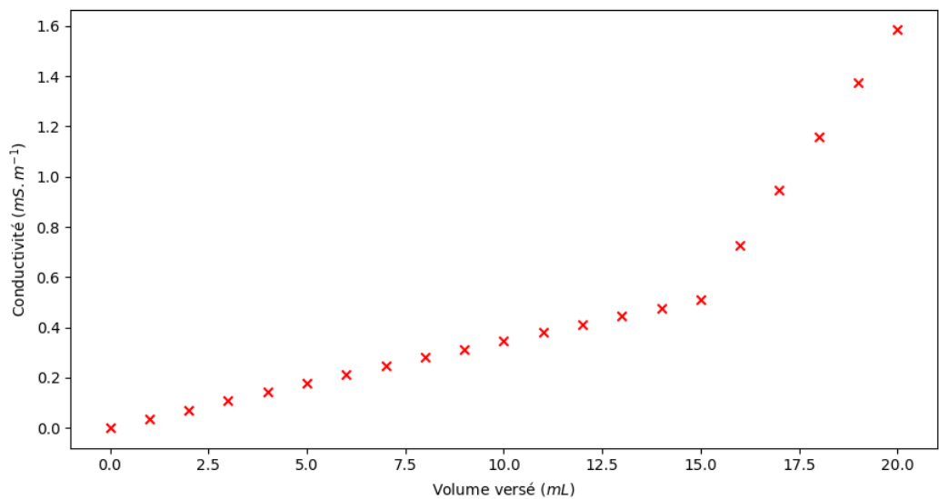
Document 3: Titrage de la solution S_1 par l'acide chlorhydrique.
