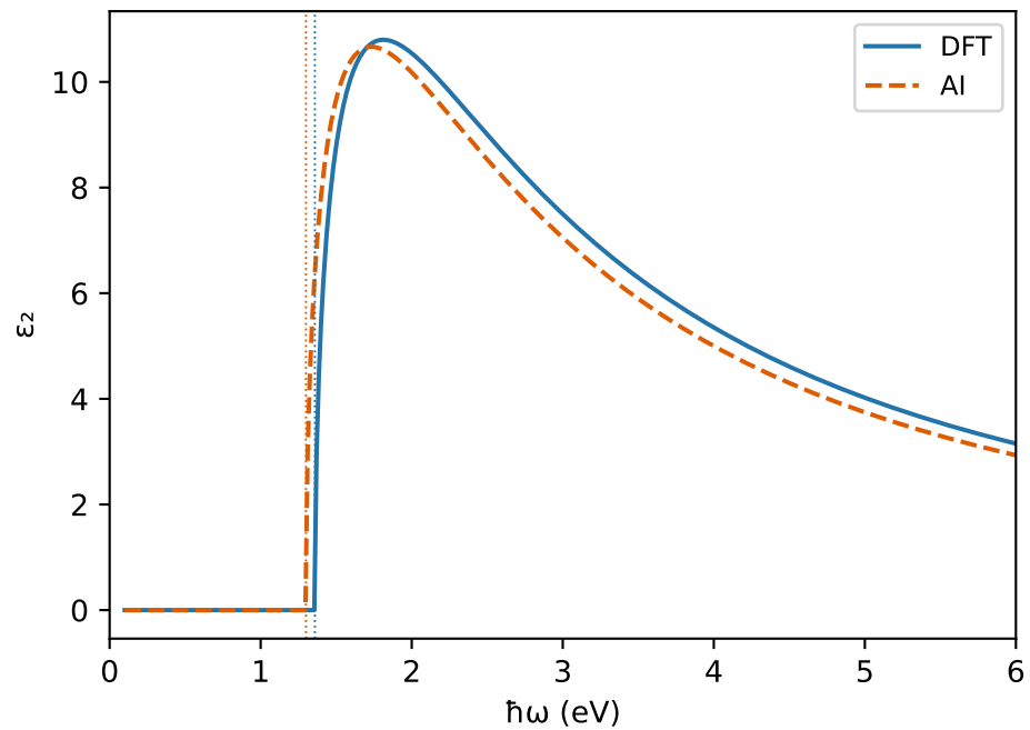
CsSnI3 — función dieléctrica DFT vs AI
