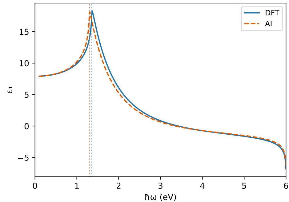
CsSnI3 — función dieléctrica DFT vs AI
