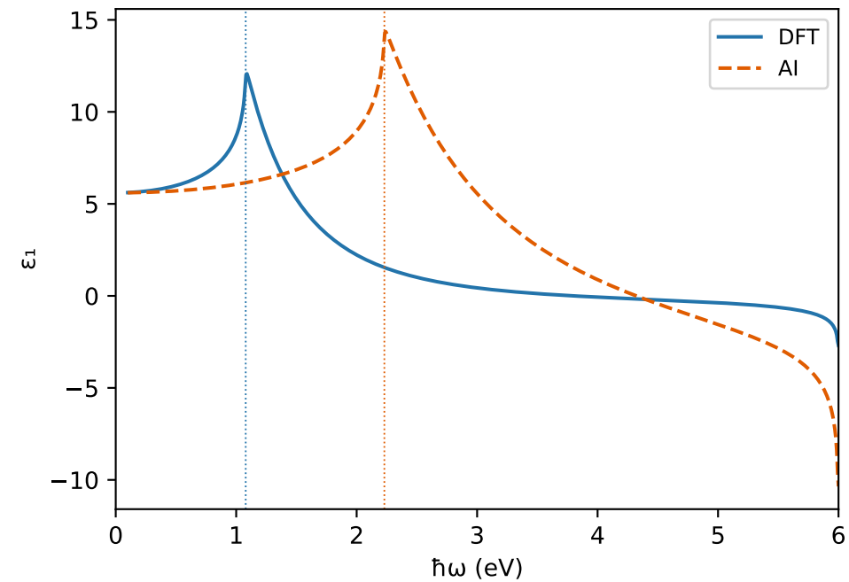
FAPbBr 3 — función dieléctrica DFT vs AI
