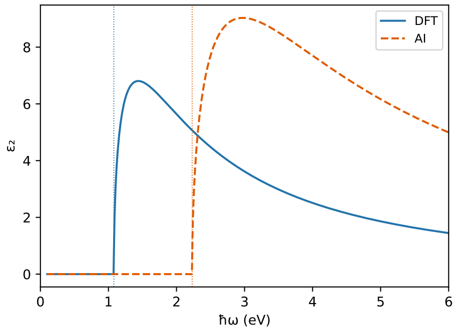
FAPbBr 3 — función dieléctrica DFT vs AI
