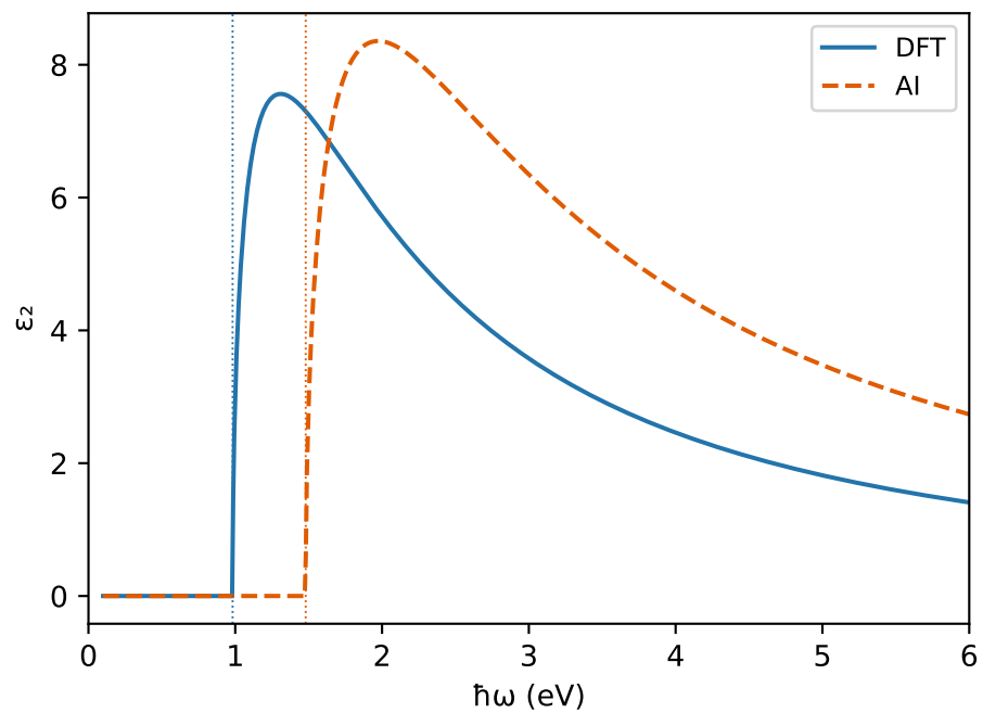
FAPbI 3 — función dieléctrica DFT vs AI
