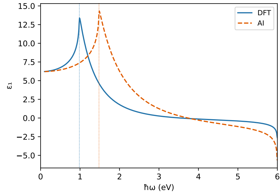
FAPbI 3 — función dieléctrica DFT vs AI
