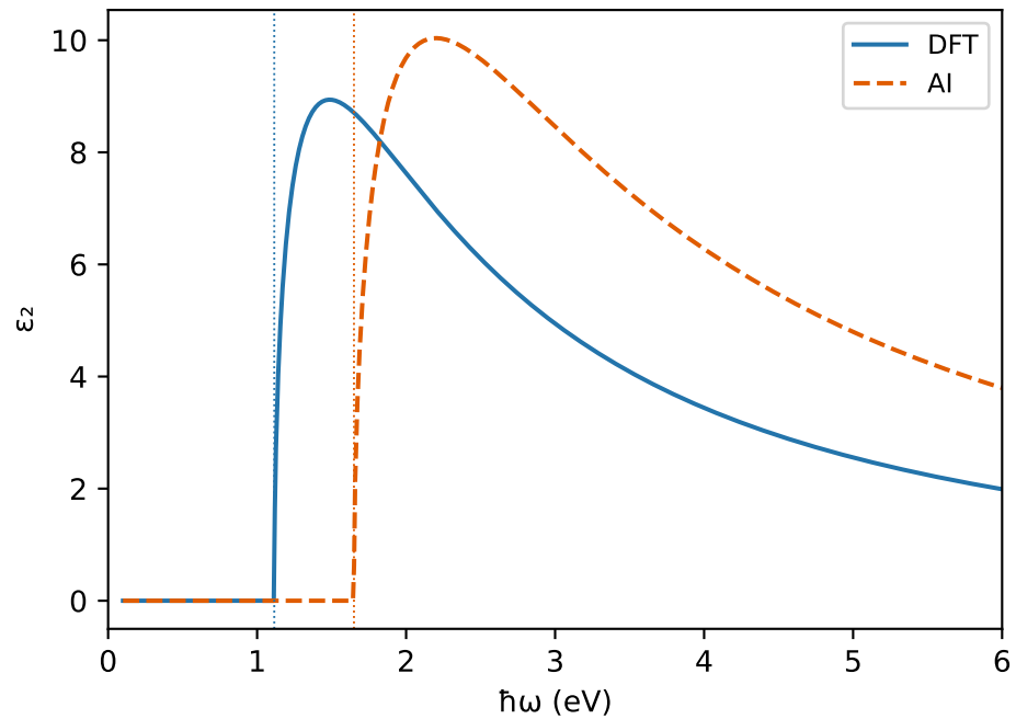
FASnBr3 — función dieléctrica DFT vs AI
