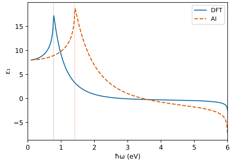
FASnI3 — función dieléctrica DFT vs AI
