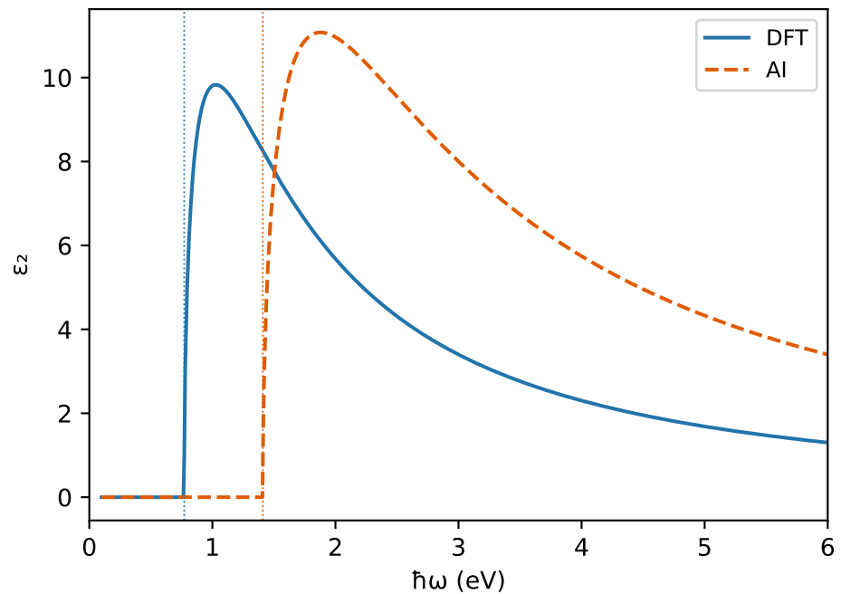
FASnI3 — función dieléctrica DFT vs AI
