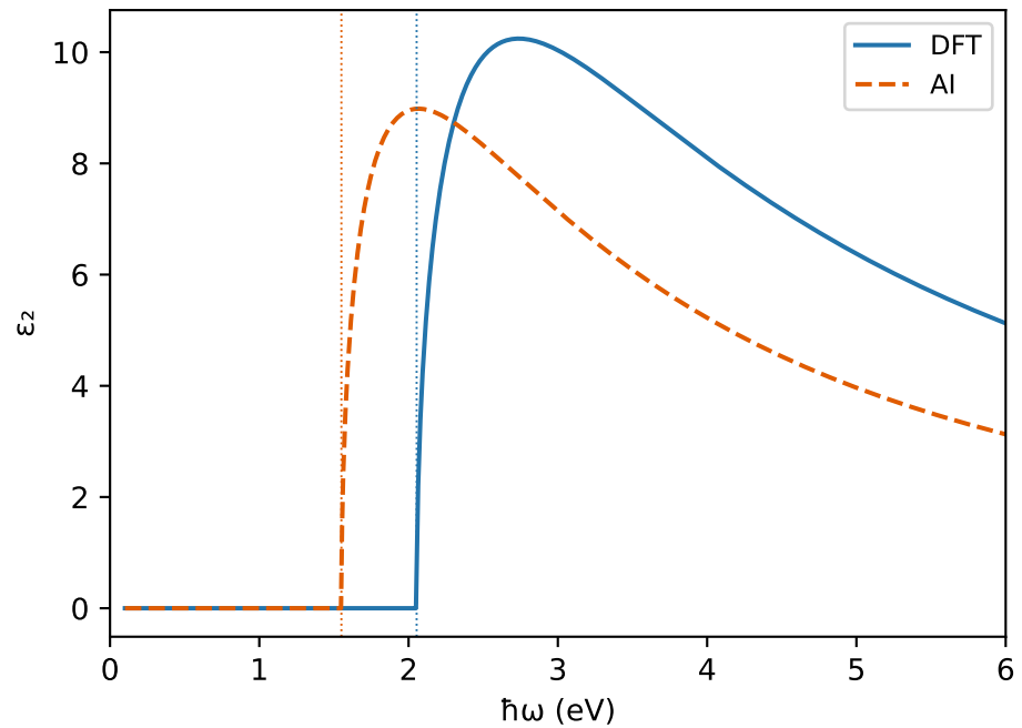
MAPbI3 — función dieléctrica DFT vs AI
