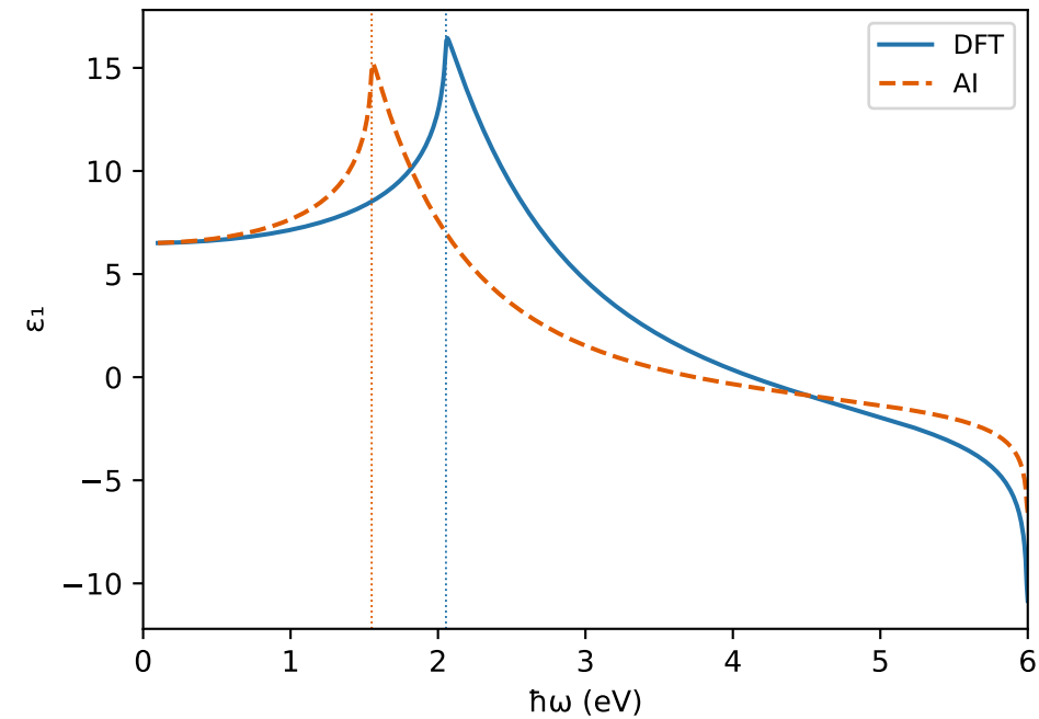
MAPbI3 — función dieléctrica DFT vs AI
