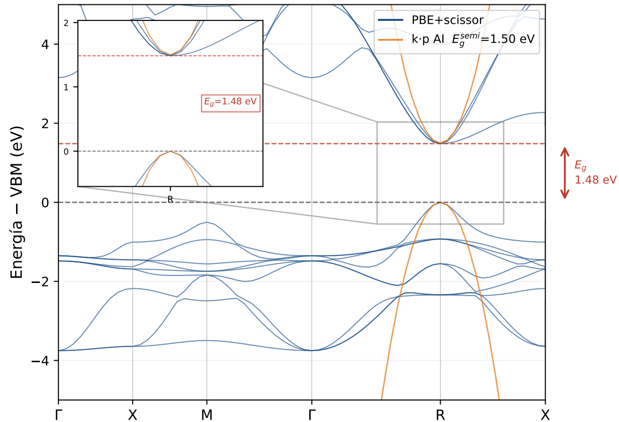
Estructura de bandas — CsPbI3 (PBE+scissor)
