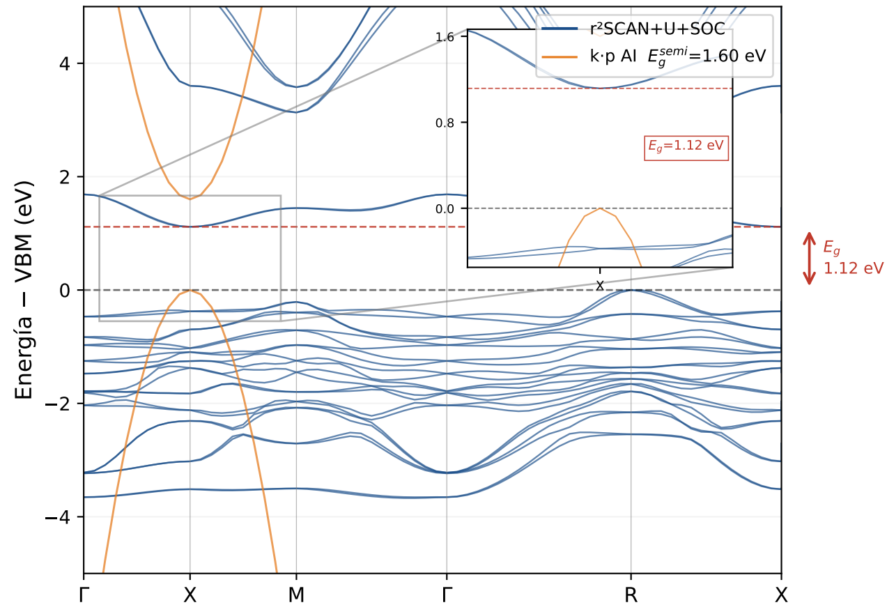
Estructura de bandas — FASnBr3 (r 2 SCAN+U+SOC)
