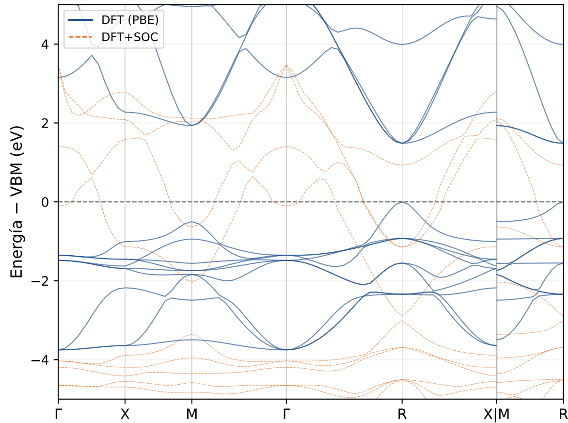
Estructura de bandas — CsPbI3 (PBE) [scissor +0.194 eV en CB]
