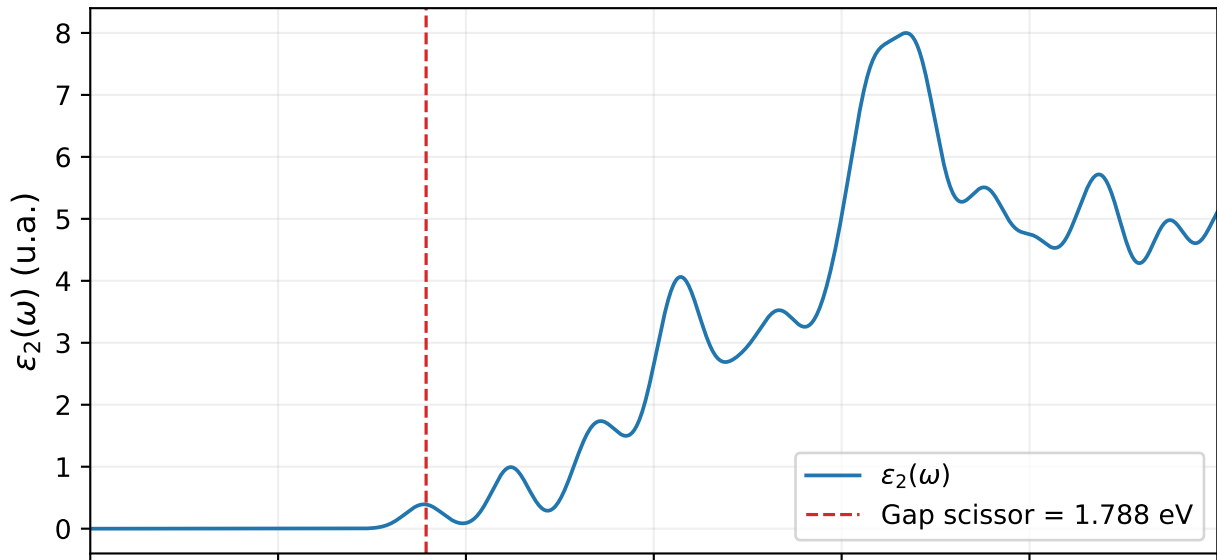
Función dieléctrica IPA — CsPbI3 [scissor +0.194 eV]
