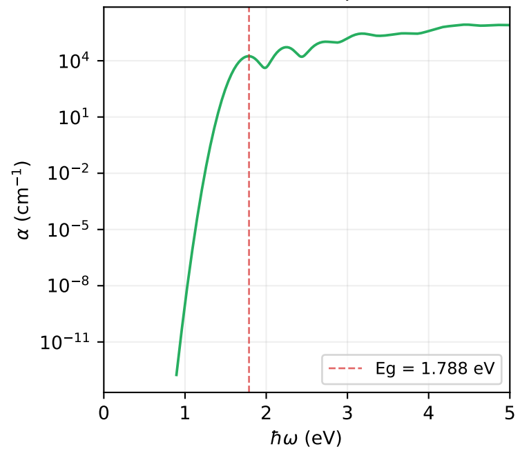
Absorción óptica
