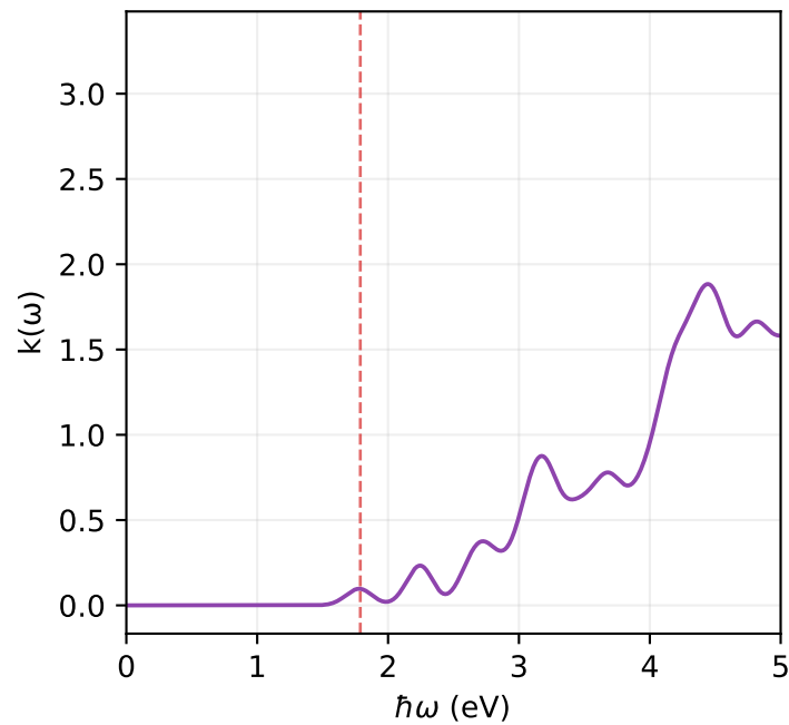
Coef. extinción
