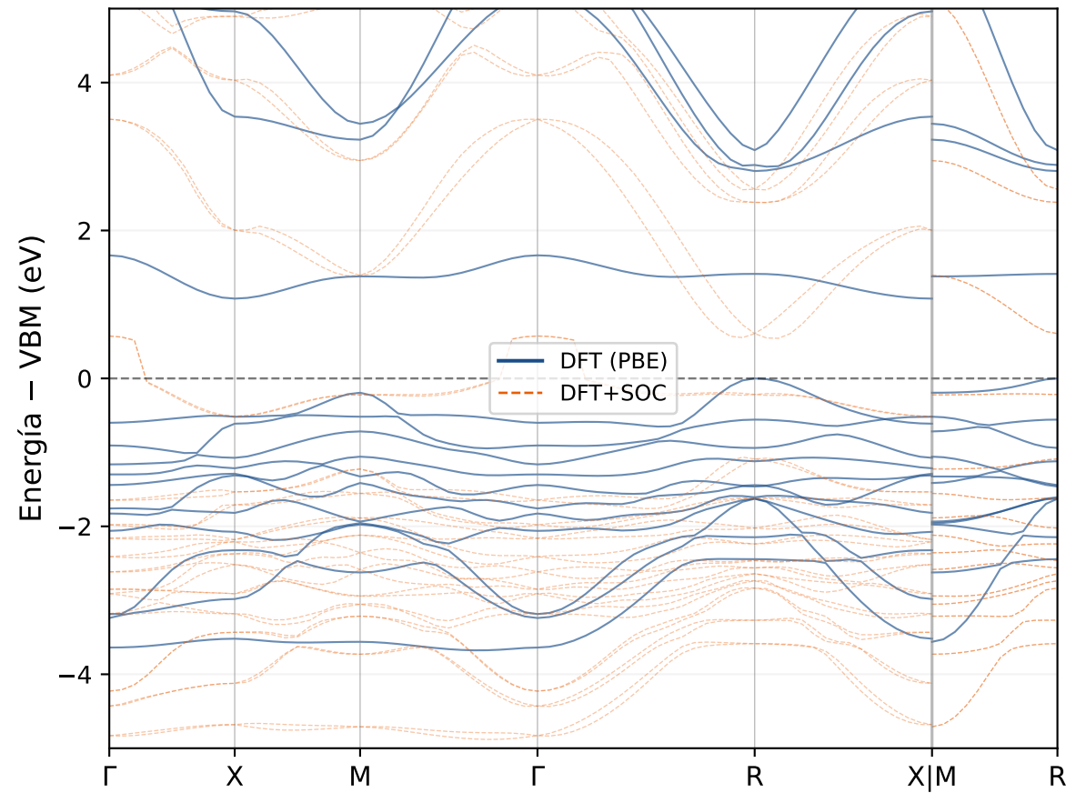
Estructura de bandas — FAPbBr 3 (PBE) [scissor +0.500 eV en CB]
