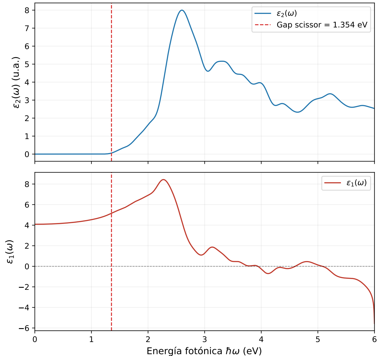
Función dieléctrica IPA — FAPbBr3 [scissor +0.500 eV]
