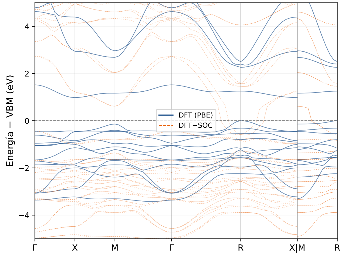
Estructura de bandas — FAPbI3 (PBE) [scissor +0.500 eV en CB]
