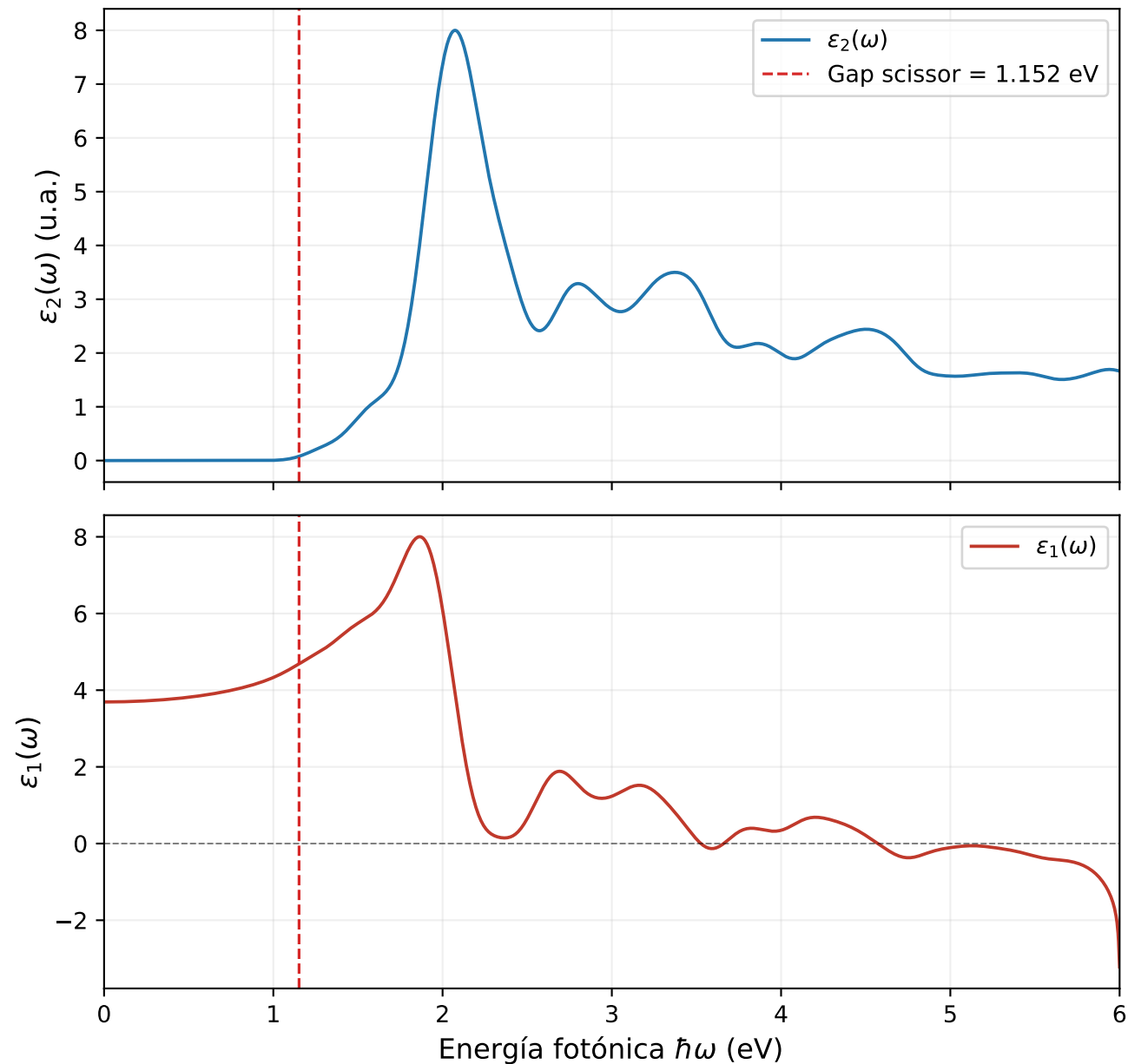
Función dieléctrica IPA — FAPbI3 [scissor +0.500 eV]
