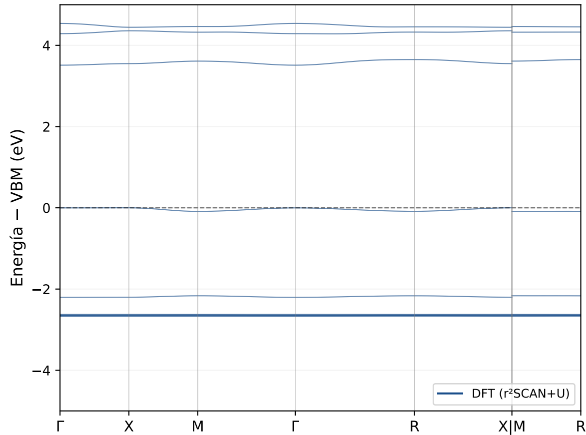
Estructura de bandas — FASnBr 3 (r 2 SCAN+U)
