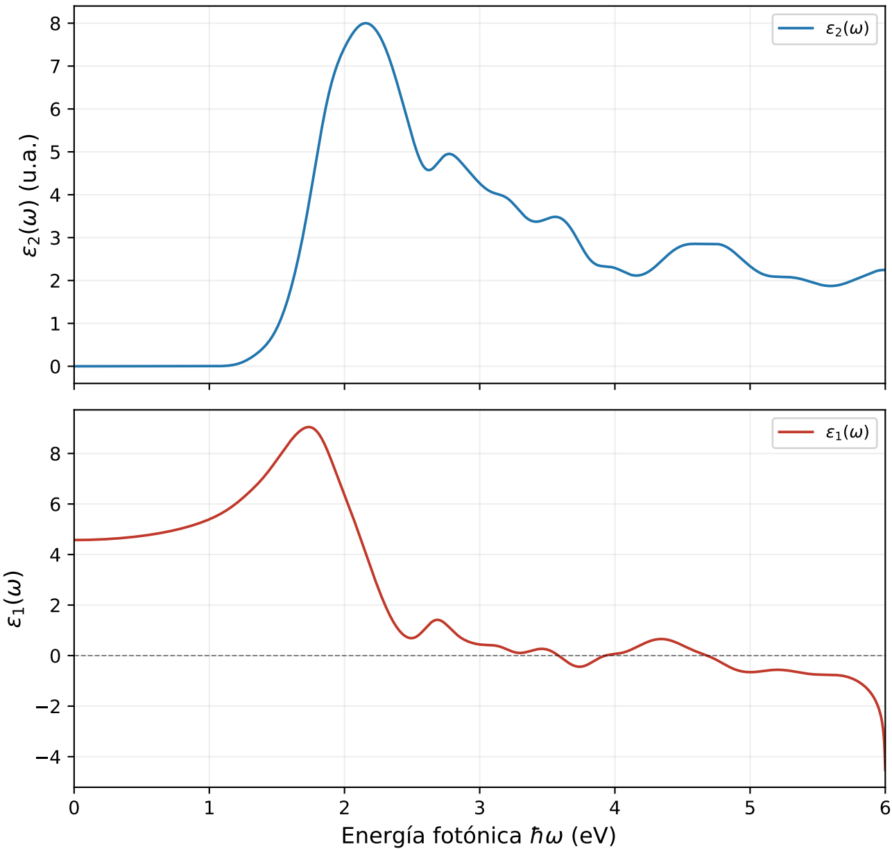
Función dieléctrica IPA — FASnBr3 [SOC gap = 1.062 eV]
