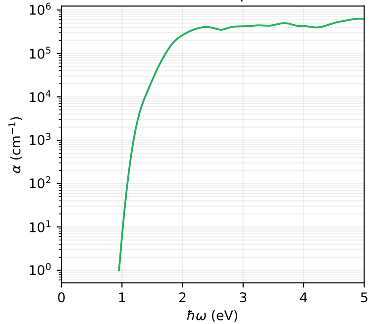
Absorción óptica
