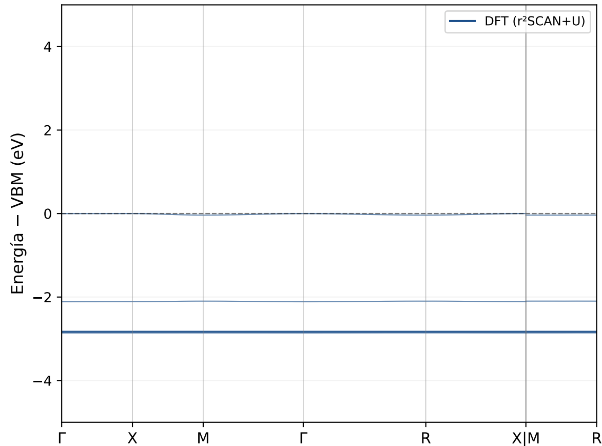
Estructura de bandas — FASnI3 (r 2 SCAN+U)
