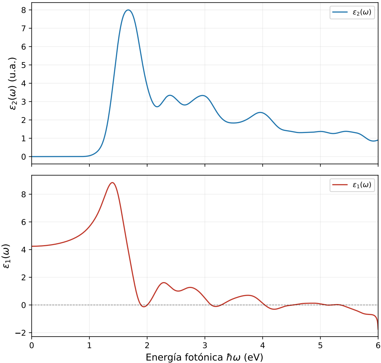
Función dieléctrica IPA — FASnI3 [SOC gap = 0.719 eV]
