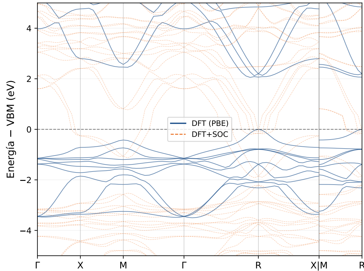
Estructura de bandas — MAPbI 3 (PBE) [scissor +0.500 eV en CB]
