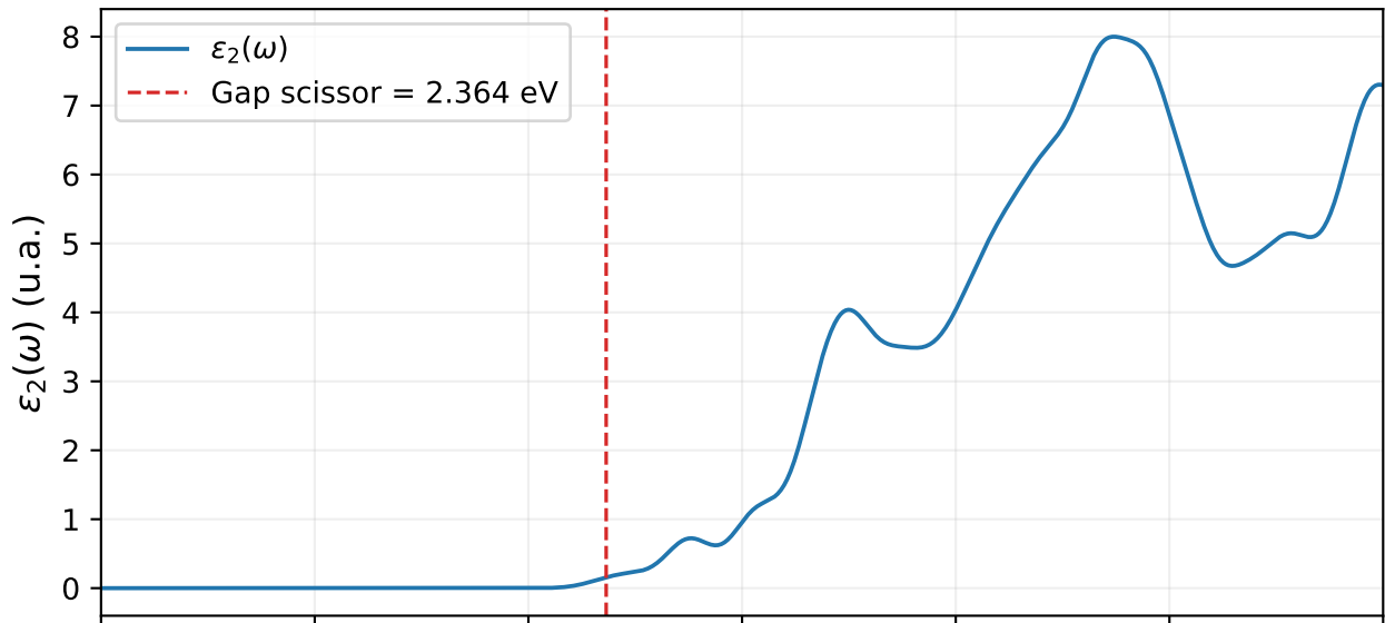
Función dieléctrica IPA — MAPbI3 [scissor +0.500 eV]
