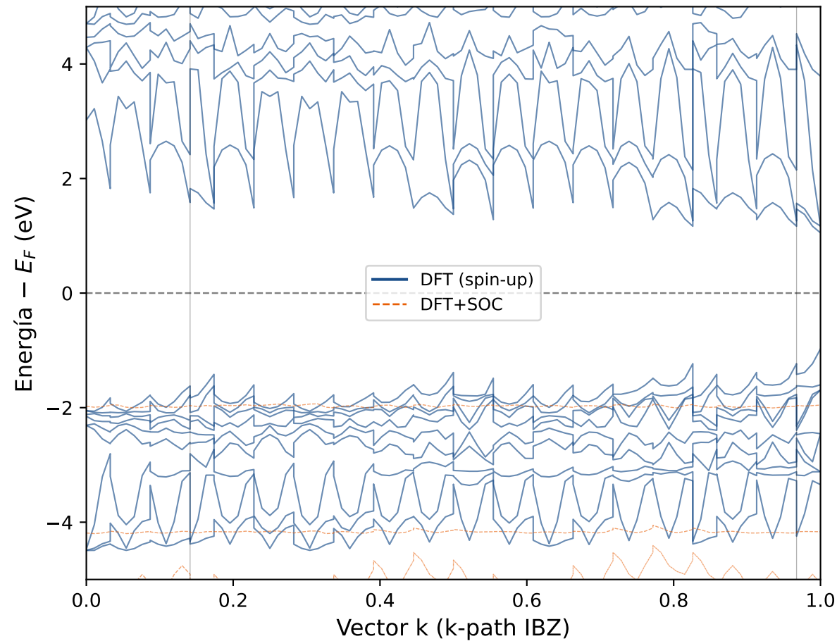
Estructura de bandas — MASnI3
