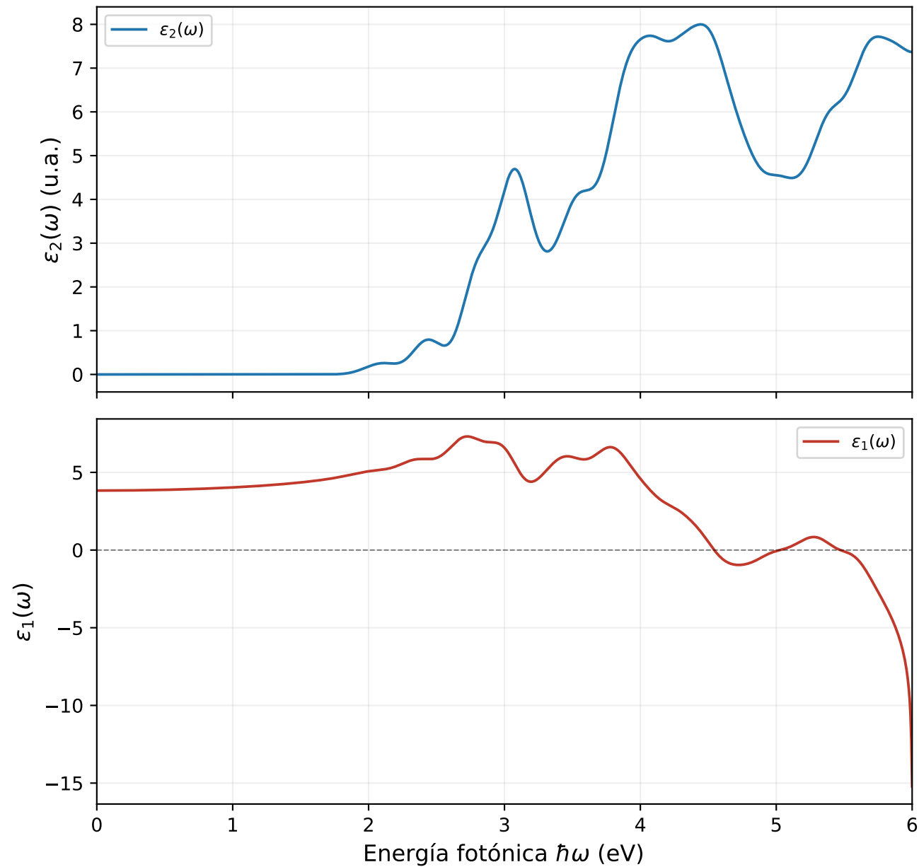
Función dieléctrica IPA — MASnI3 [SOC gap = 1.593 eV]
