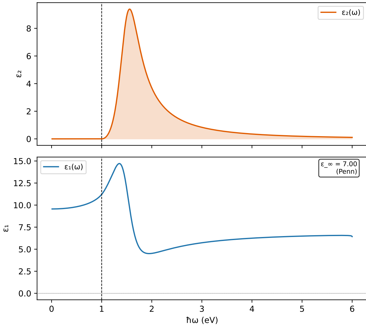
CsPbI3 — Función dieléctrica AI (Tauc-Lorentz)
