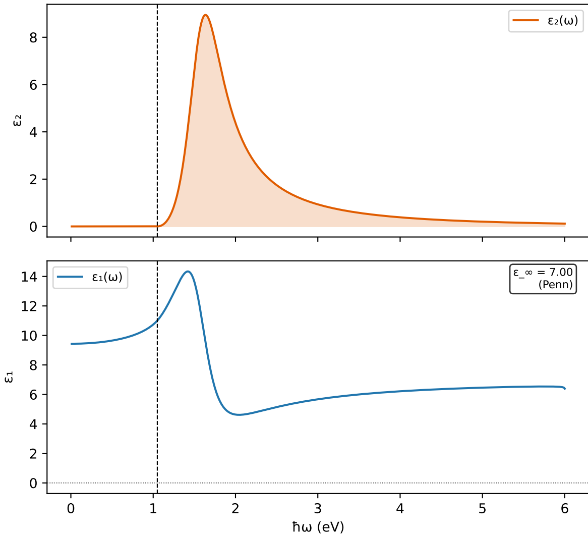
CsSnI3 — Función dieléctrica AI (Tauc-Lorentz)
