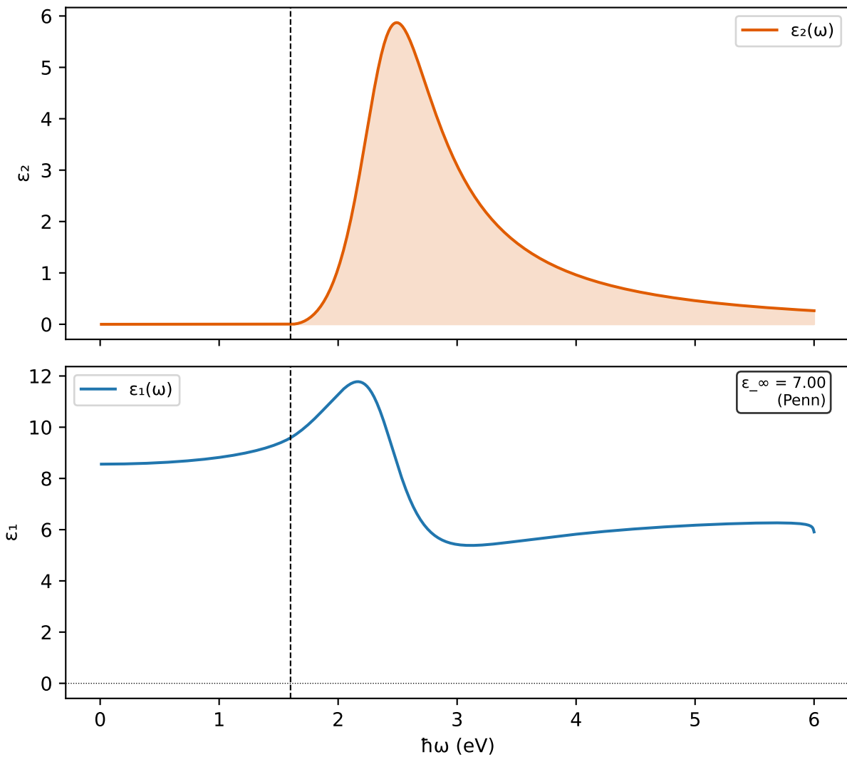
FAPbBr3 — Función dieléctrica AI (Tauc-Lorentz)
