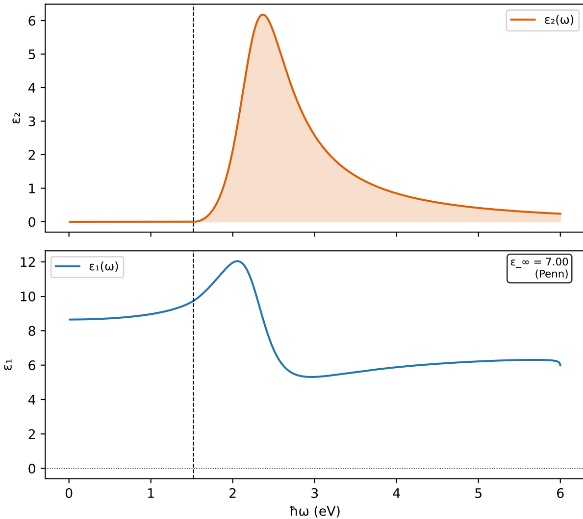
FASnBr3 — Función dieléctrica AI (Tauc-Lorentz)
