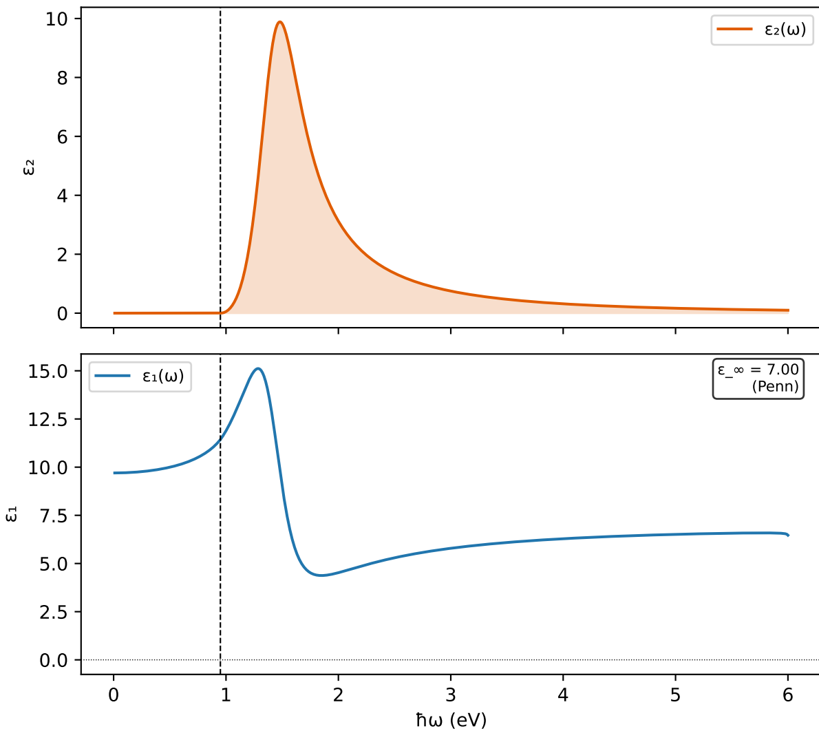
MAPbI3 — Función dieléctrica AI (Tauc-Lorentz)
