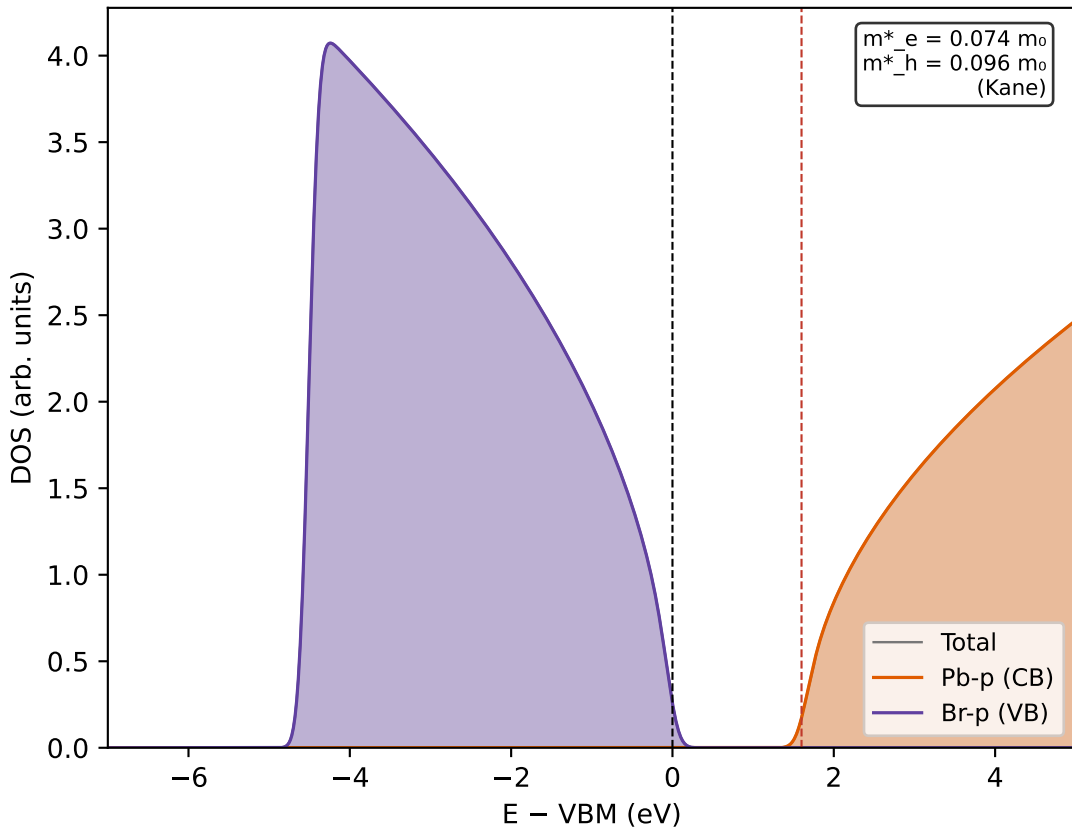
FAPbBr3 — DOS AI (3D parabólica)
