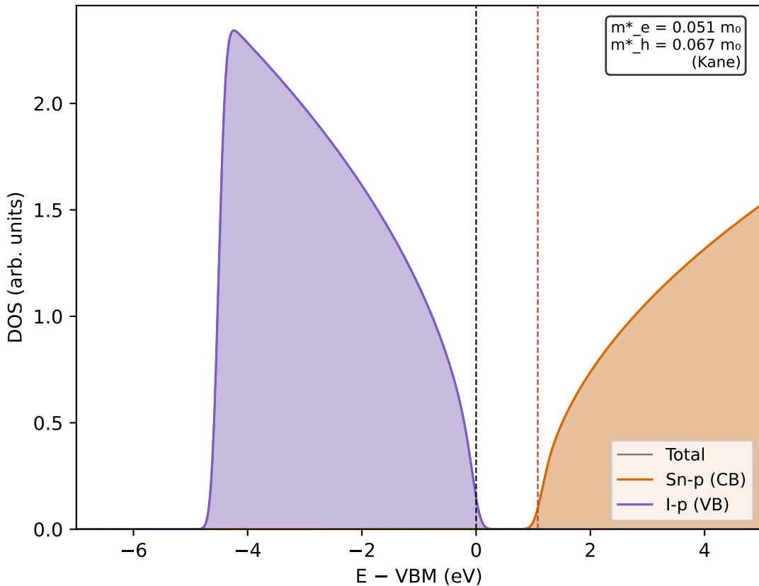
MASnI3 — DOS AI (3D parabólica)
