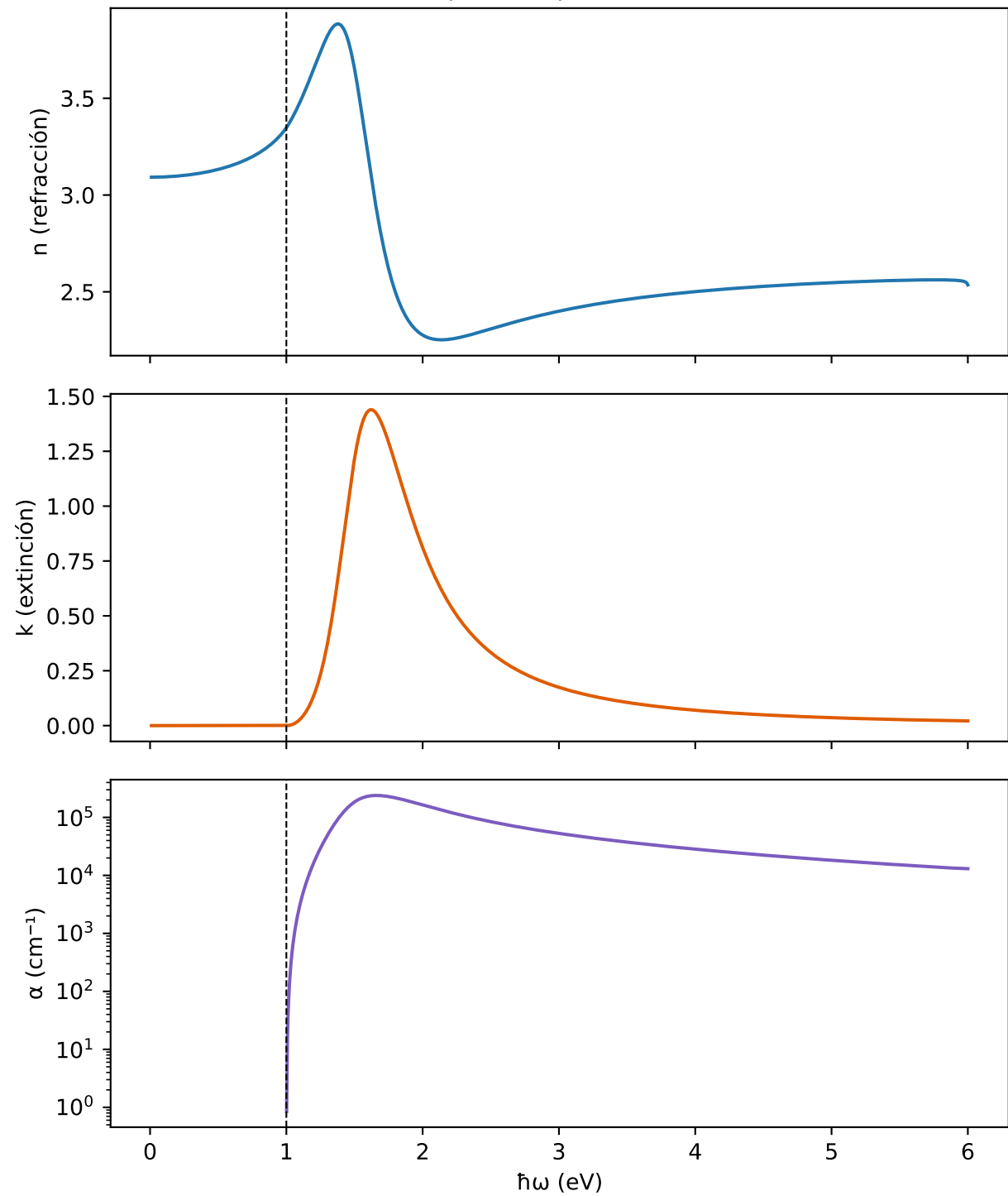
CsPbI3 — Espectro óptico AI (Tauc-Lorentz)
