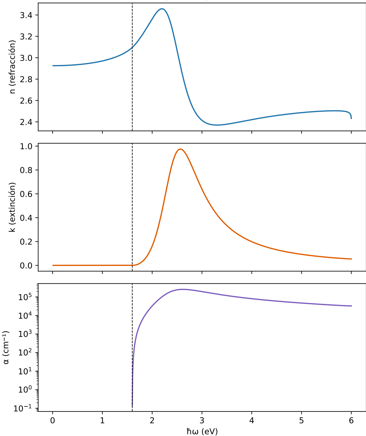
FAPbBr3 — Espectro óptico AI (Tauc-Lorentz)
