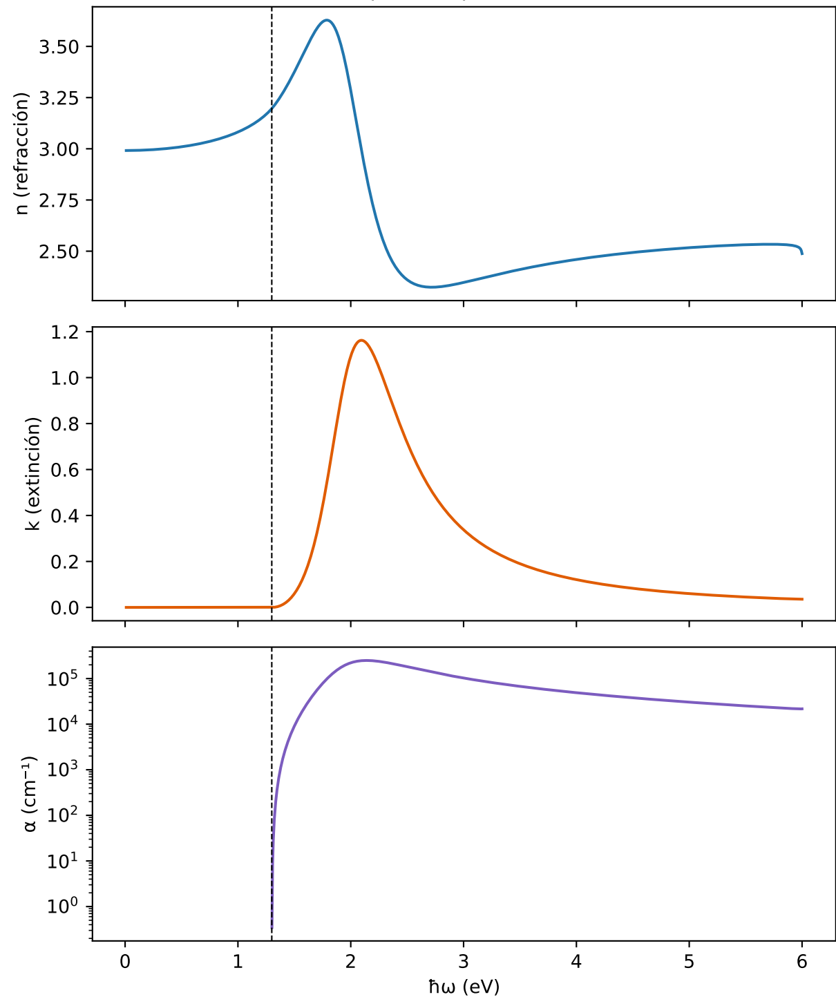
FAPbI3 — Espectro óptico AI (Tauc-Lorentz)
