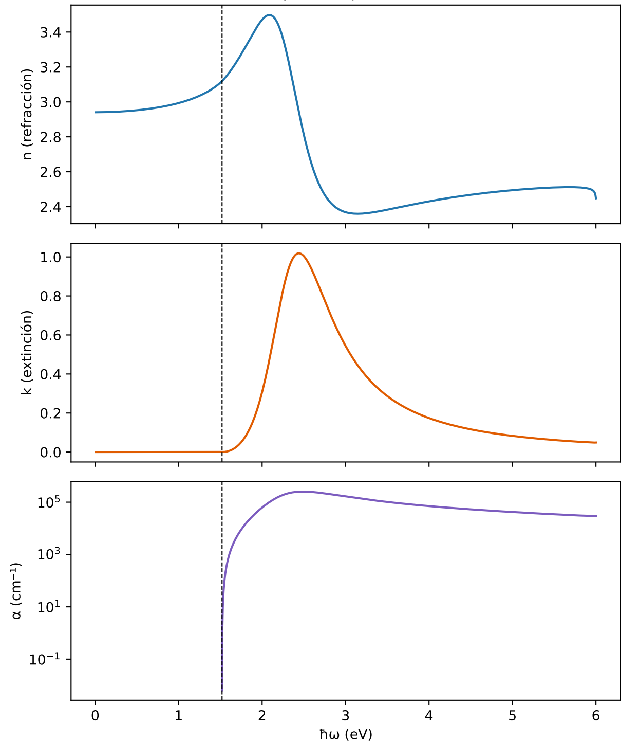
FASnBr3 — Espectro óptico AI (Tauc-Lorentz)
