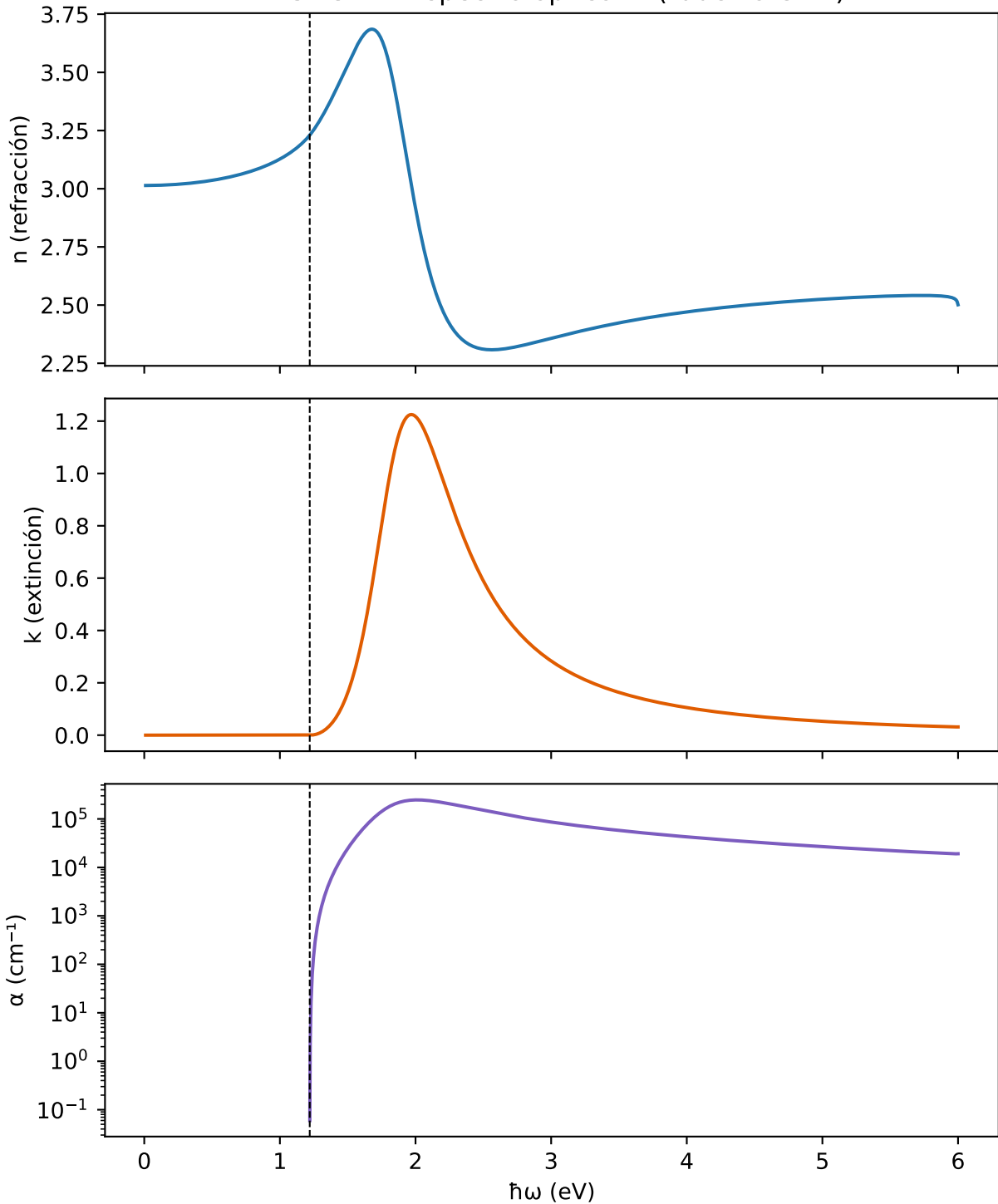
FASnI3 — Espectro óptico Al (Tauc-Lorentz)
