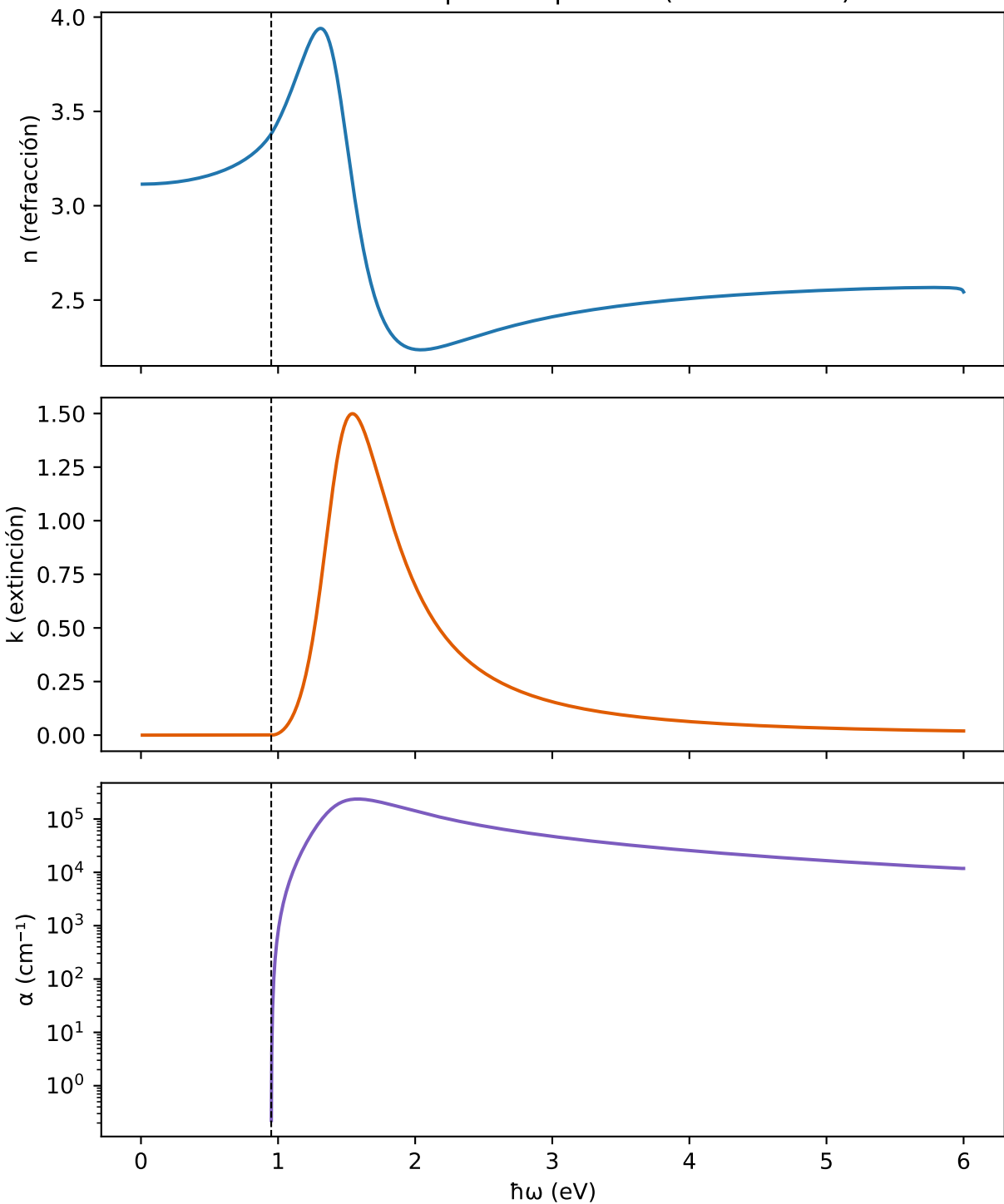
MAPbI3 — Espectro óptico AI (Tauc-Lorentz)
