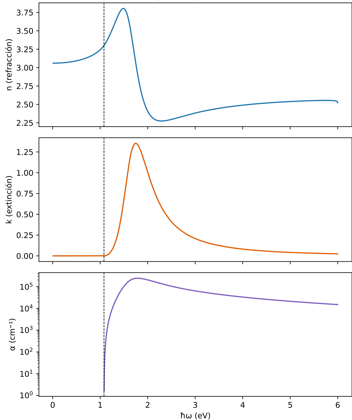
MASnI3 — Espectro óptico Al (Tauc-Lorentz)
